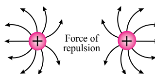
Fig: 14.11 (d) Two equal like charges
