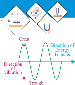
Fig: 10.7 Transverse wave
