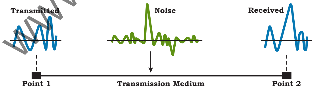
Fig: 4.14 Noise
