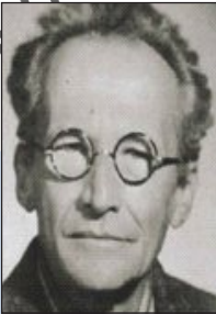
شکل 2.15 شرڈنگر
