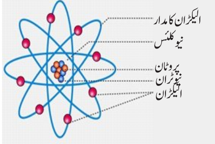
شکل 2.12 رد فورڈ ایٹمی ماڈل
