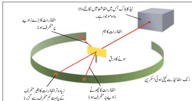
شکل 2.10 گولڈ فویل تجربہ
