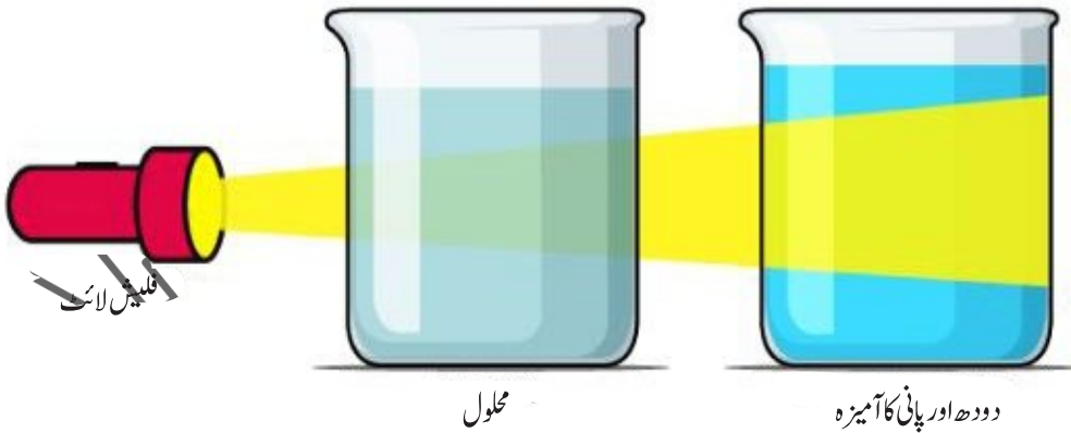
شکل 6.4 کولائیڈ کا ٹائڈل اثر
