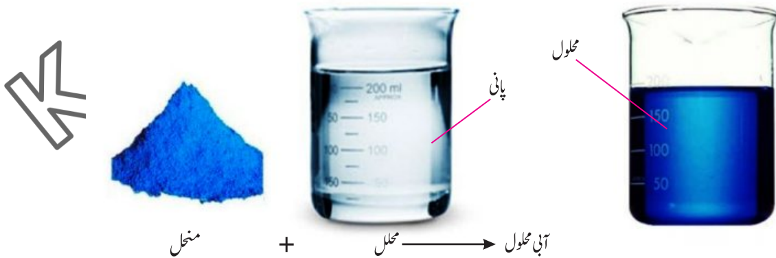
شکل 6.1 محلول کی تیاری
