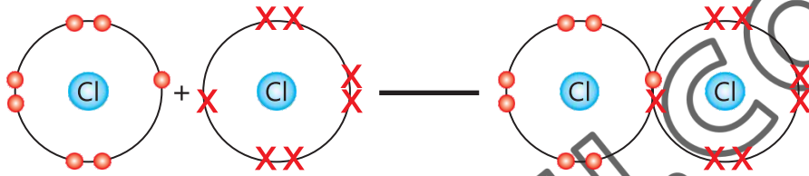
شکل 4.5 کلورین کے سالے میں واحد کوویلنٹ بونڈ کا بننا
