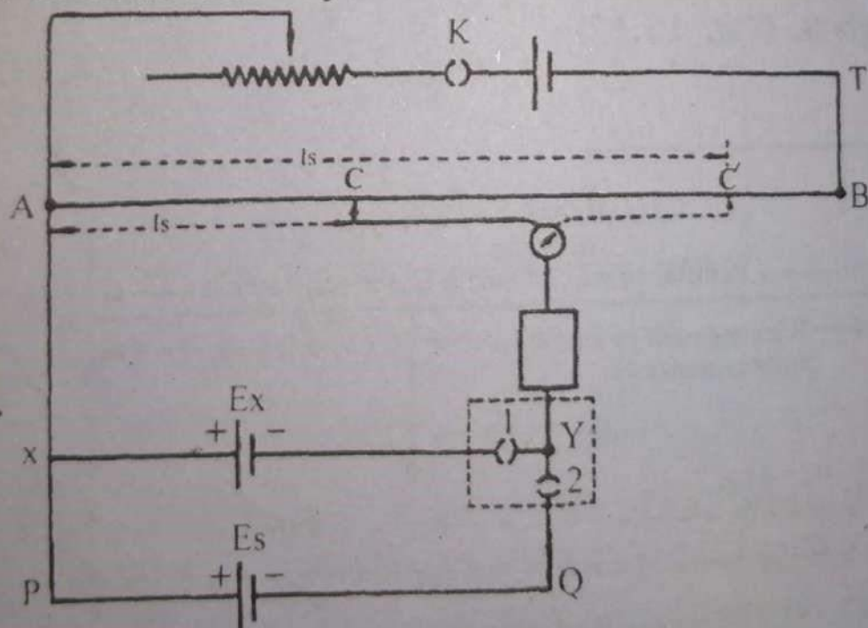
Fig. 15.13 A Potentiometer
